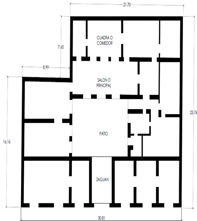
PRIMER NIVEL
