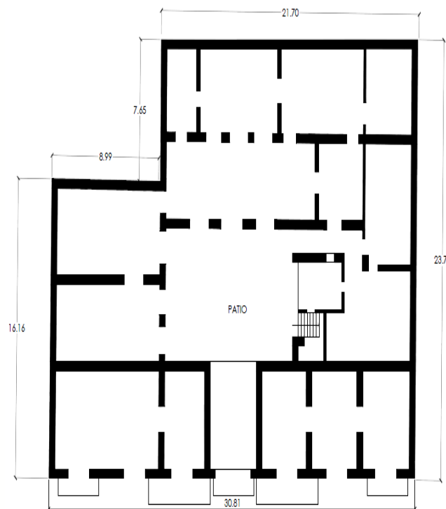
SEGUNDO NIVEL
